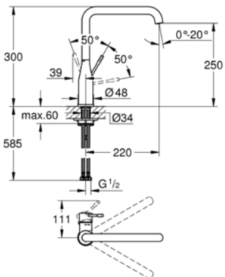
30 372 000 Essence sink mixer
