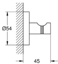
40 364 EN1 40 364 A01 40 364 GN1 Robe hook
