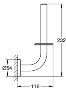
40 385 001 Spare toilet roll holder
