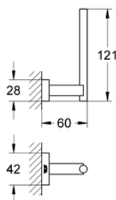
40 623 001 Spare toilet roll holder
