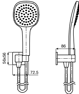
Bloc Handshower
