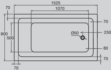
Domaine Inset Bath
