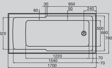
Domaine Shower Bath
