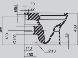
Domaine Rimless Toilet Pan
