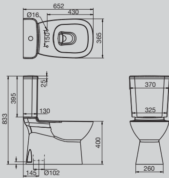
Domaine Close Coupled Rimless Toilet Suite
